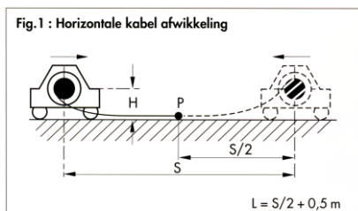
Haspel op het bewegend apparaat, Kabel met op de grond of op ondersteuningspunten
